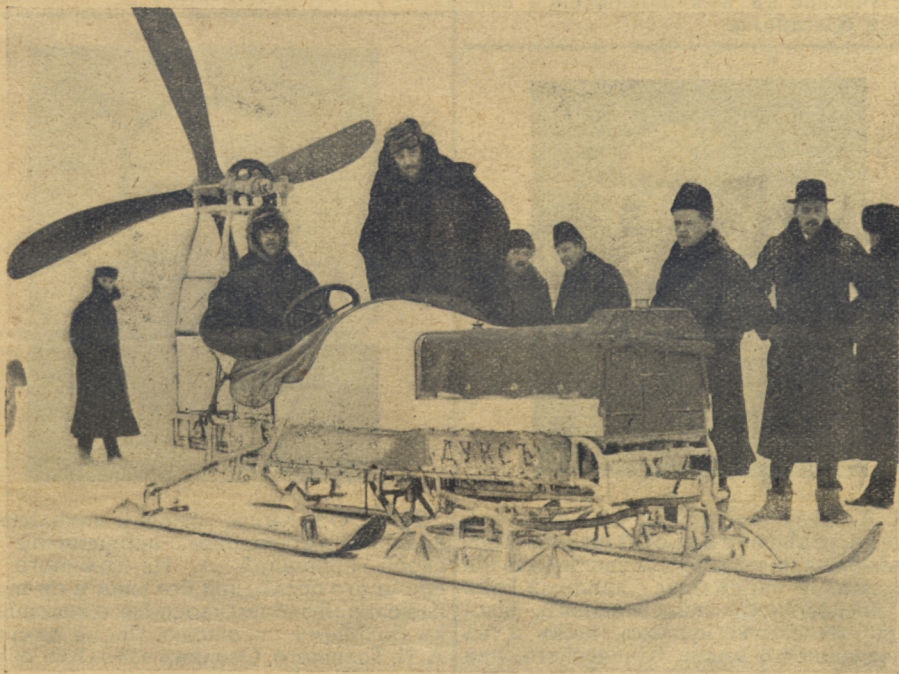
Аэро-сани завода «Духъ» Меллера.
